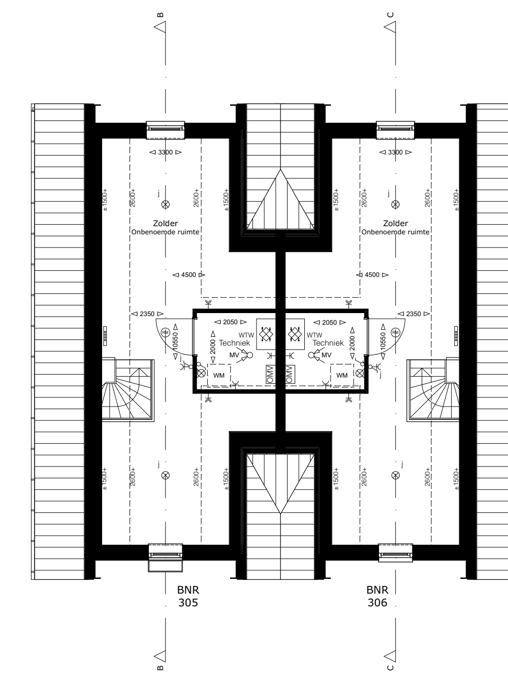
2e verdieping
