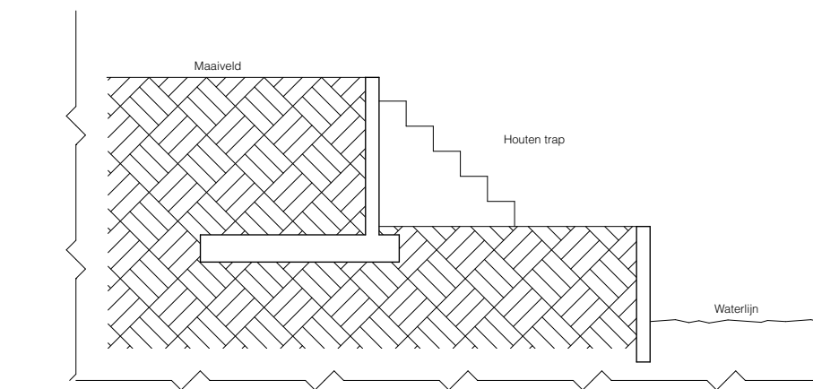
Doorsnede E-E
