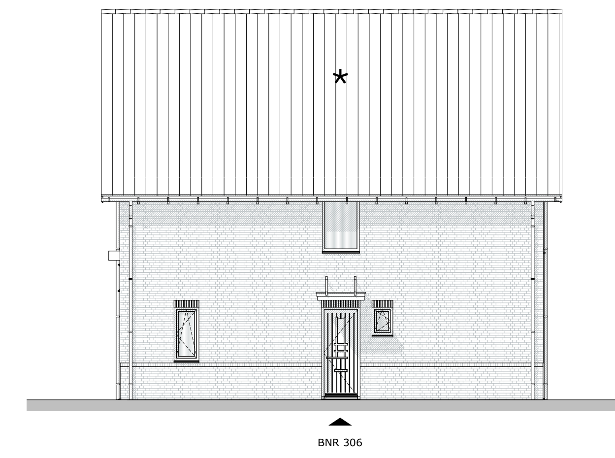
Rechterzijgevel
