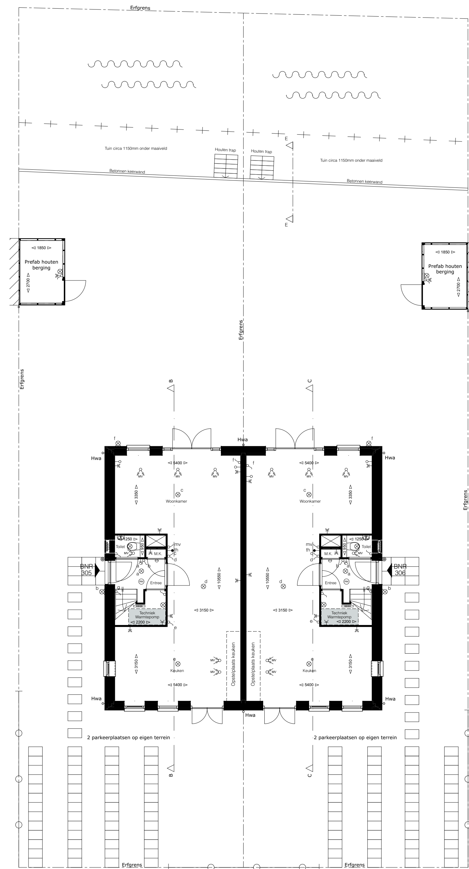
Begane grond
