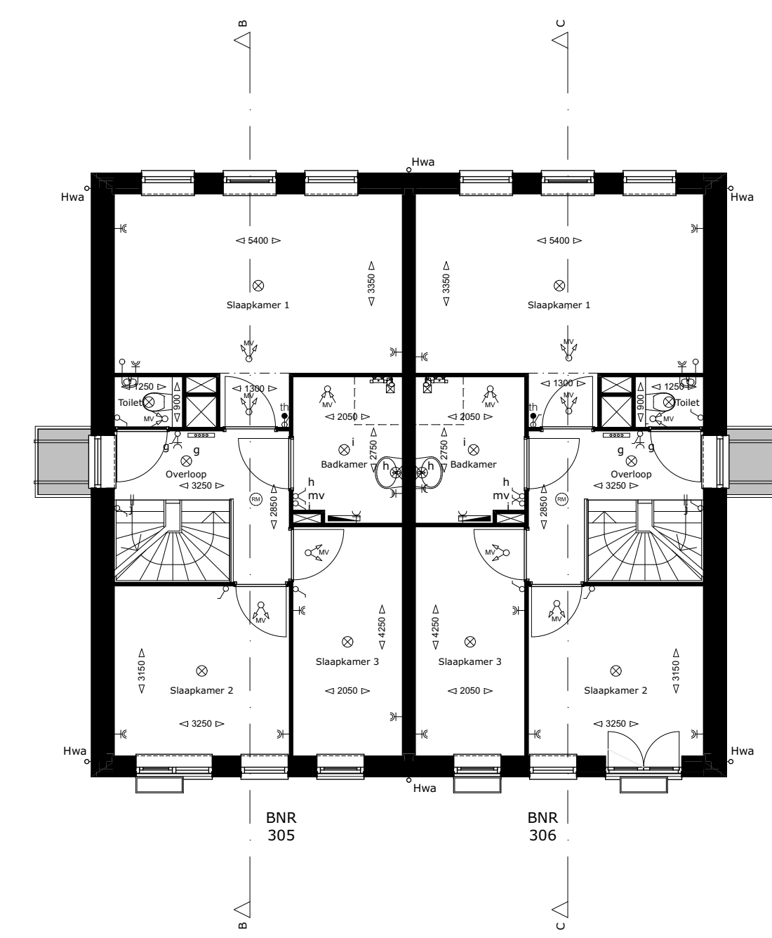
1e verdieping
