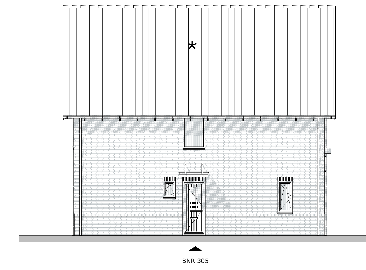
Linkerzijgevel
