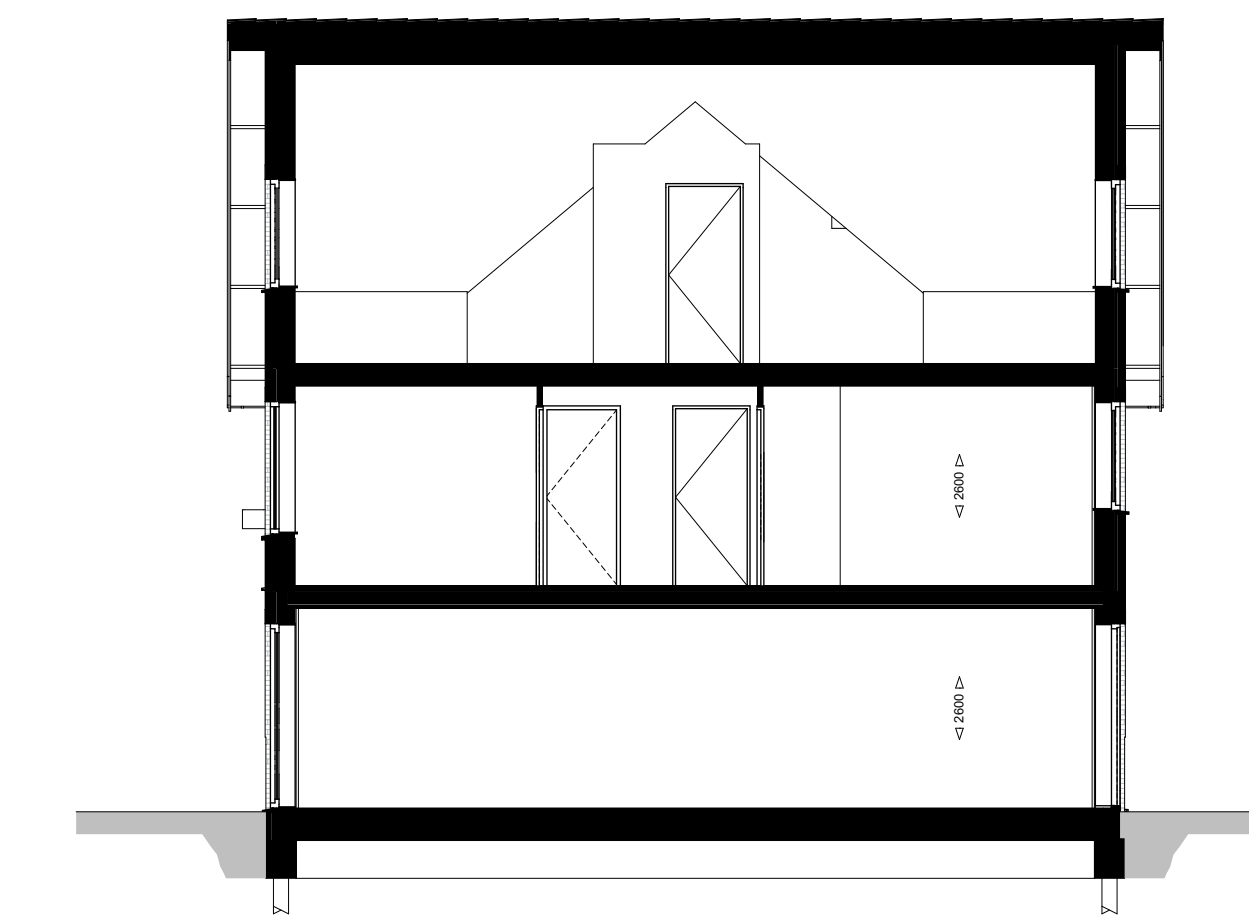
Doorsnede C-C
