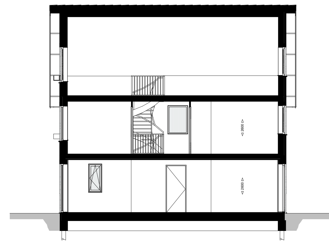
Doorsnede B-B
